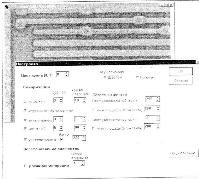
Рис. 4. Главное окно подсистемы предварительной обработки
