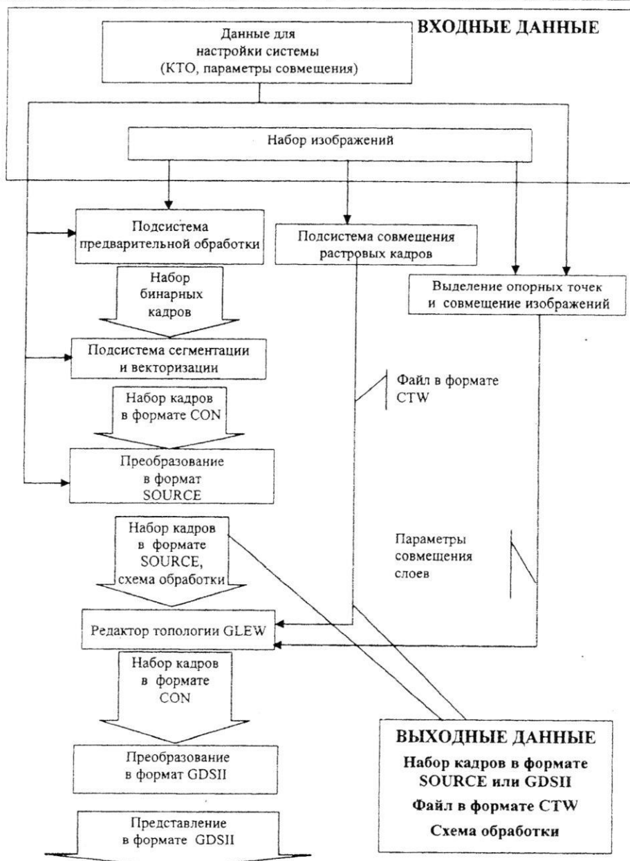
Рис. 1. Схема обработки изображений топологических слоев ИС на одной ПЭВМ
